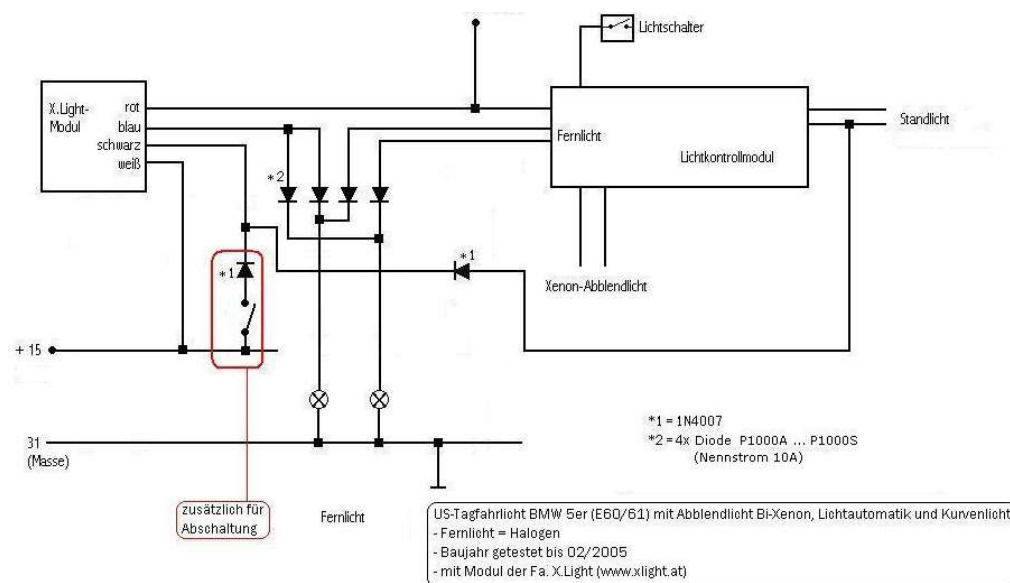
Schaltplan BMW Tagfahrlicht
